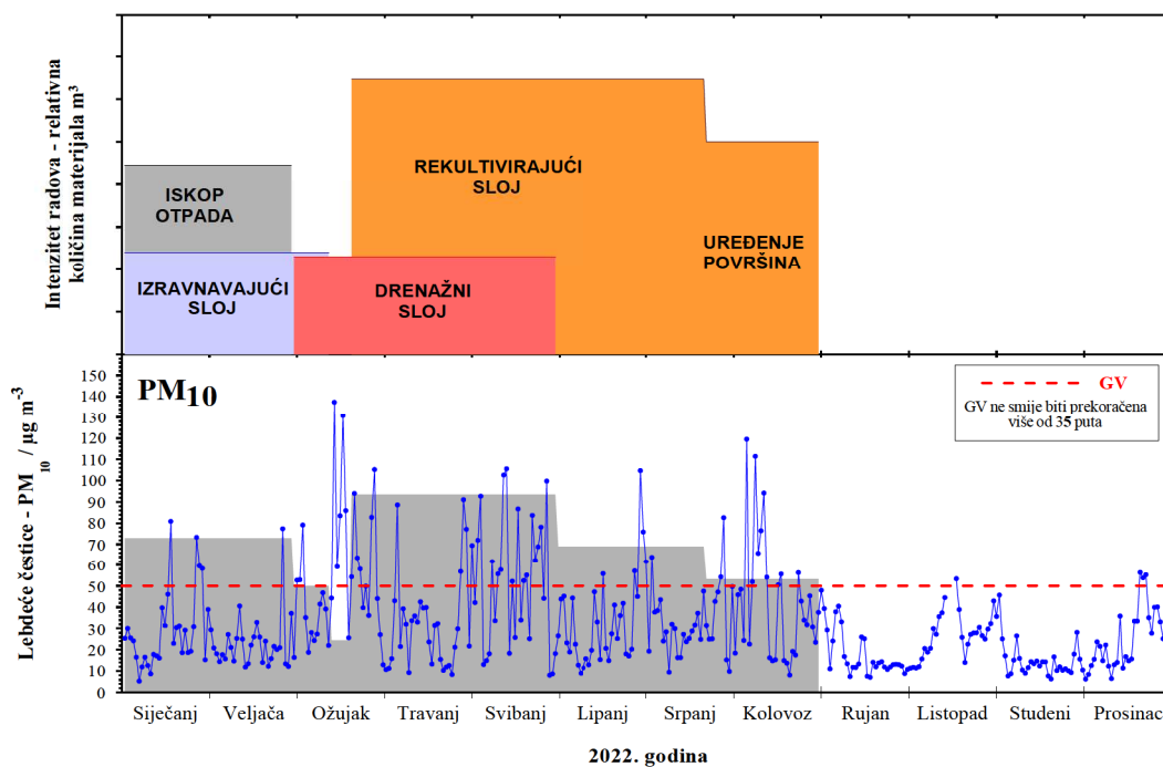
Slika 6. Prikaz mjerenja lebdećih čestica na mjestnoj postaji ŽGCO Kaštijun uz prikaz intenziteta radova na sanaciji starog odlagališta Kaštijun u 2022. godini
