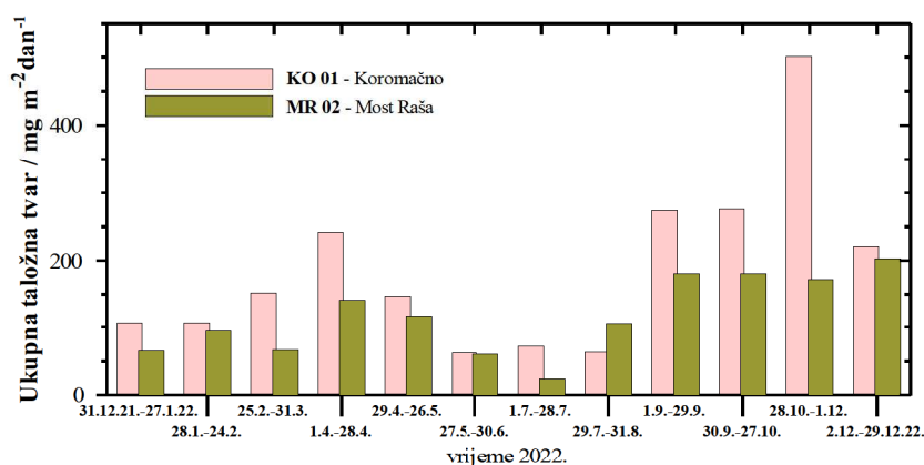
Slika 5. Kretanje mjesečnih količina ukupnih taložnih tvari u 2022. godini
