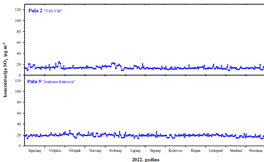
Slika 1. Kretanje srednjih dnevnih koncentracija sumporova dioksida na području Grada Pule u 2022. godini
