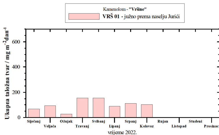
Slika 7. Kretanje mjesečnih količina ukupnih taložnih tvari za razdoblje u 2022. godini
