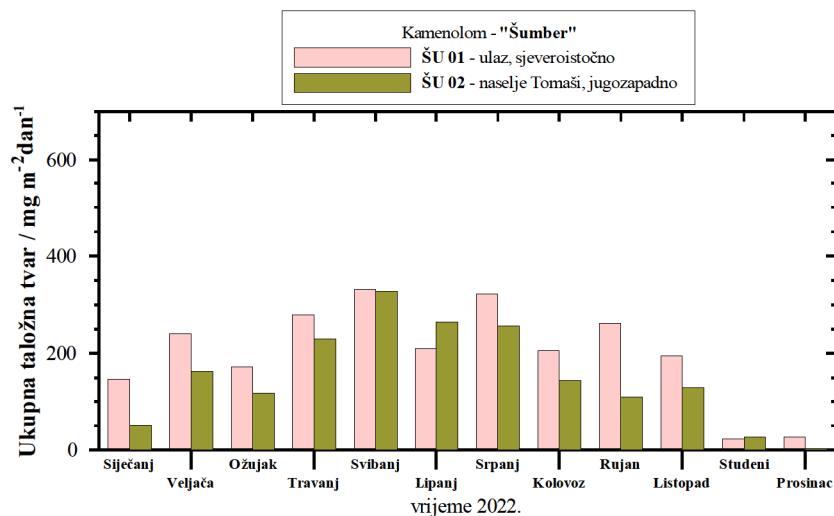
Slika 9. Kretanje mjesečnih količina ukupnih taložnih tvari za razdoblje u 2022. godini
