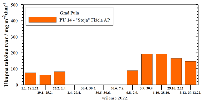
Slika 4. Kretanje mjesečnih količina ukupnih taložnih tvari za razdoblje u 2022. godini
