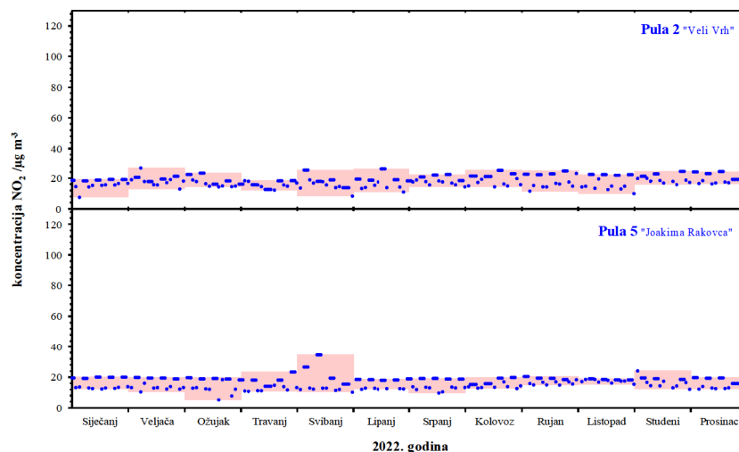
Slika 3. Kretanje srednjih dnevnih koncentracija dušikova dioksida na području Grada Pule u 2022. godini
