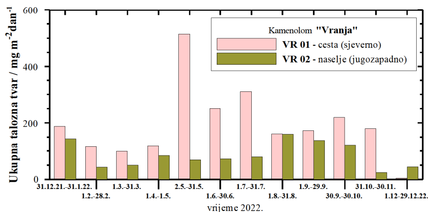
Slika 8. Kretanje mjesečnih količina ukupnih taložnih tvari za razdoblje u 2022. godini
