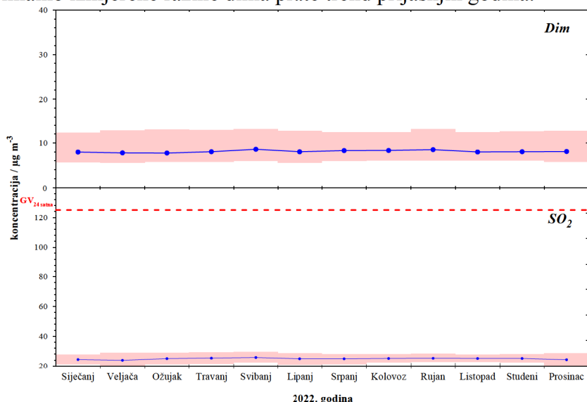
Slika 2. Kretanje srednjih dnevnih koncentracija sumporova dioksida i dima na području Općine Raša u 2022. godini
