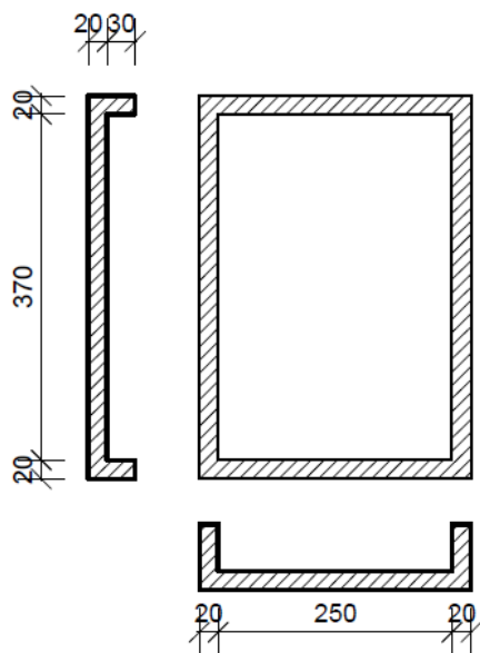
TANKVANA 5 250/370/30 cm
