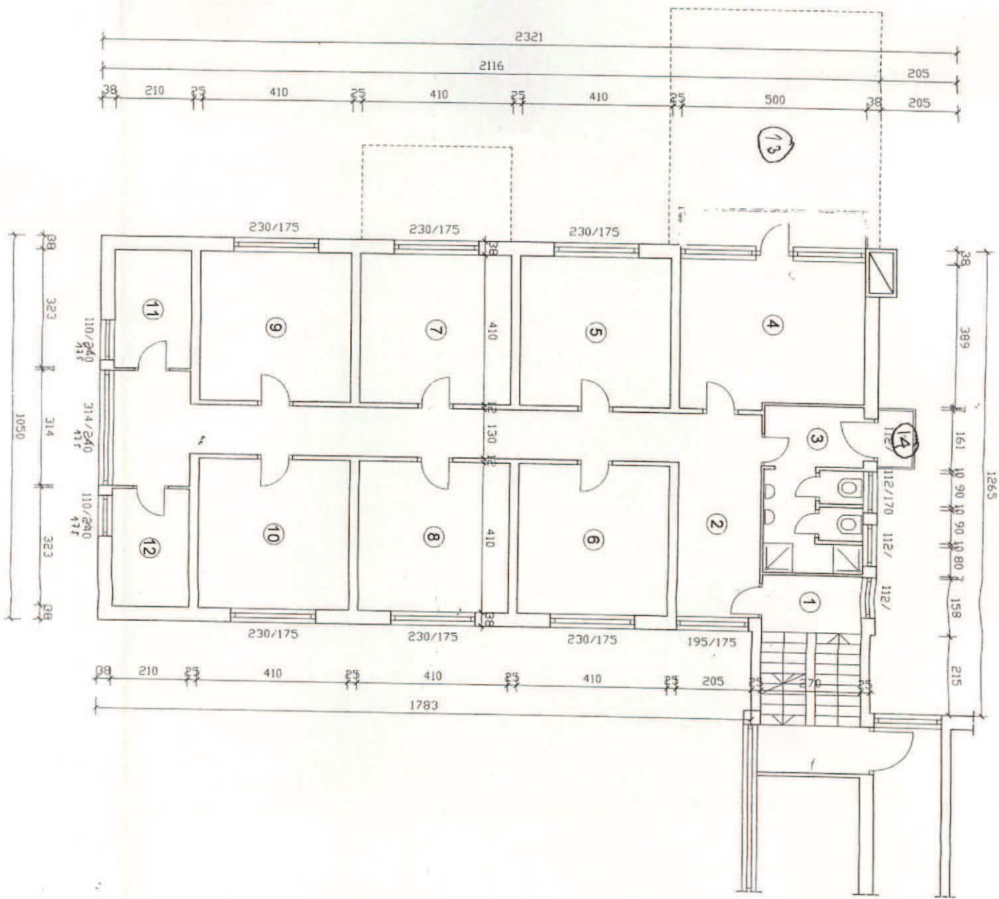
Postojeće stanje Tlocrt 1. kata M1:100
