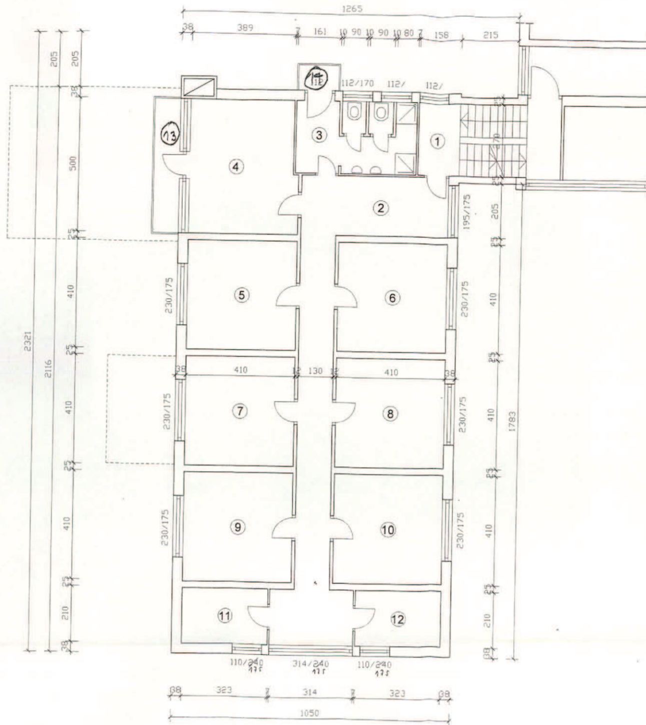
Postojeće stanje Tlocrt 2. kata M1:100
