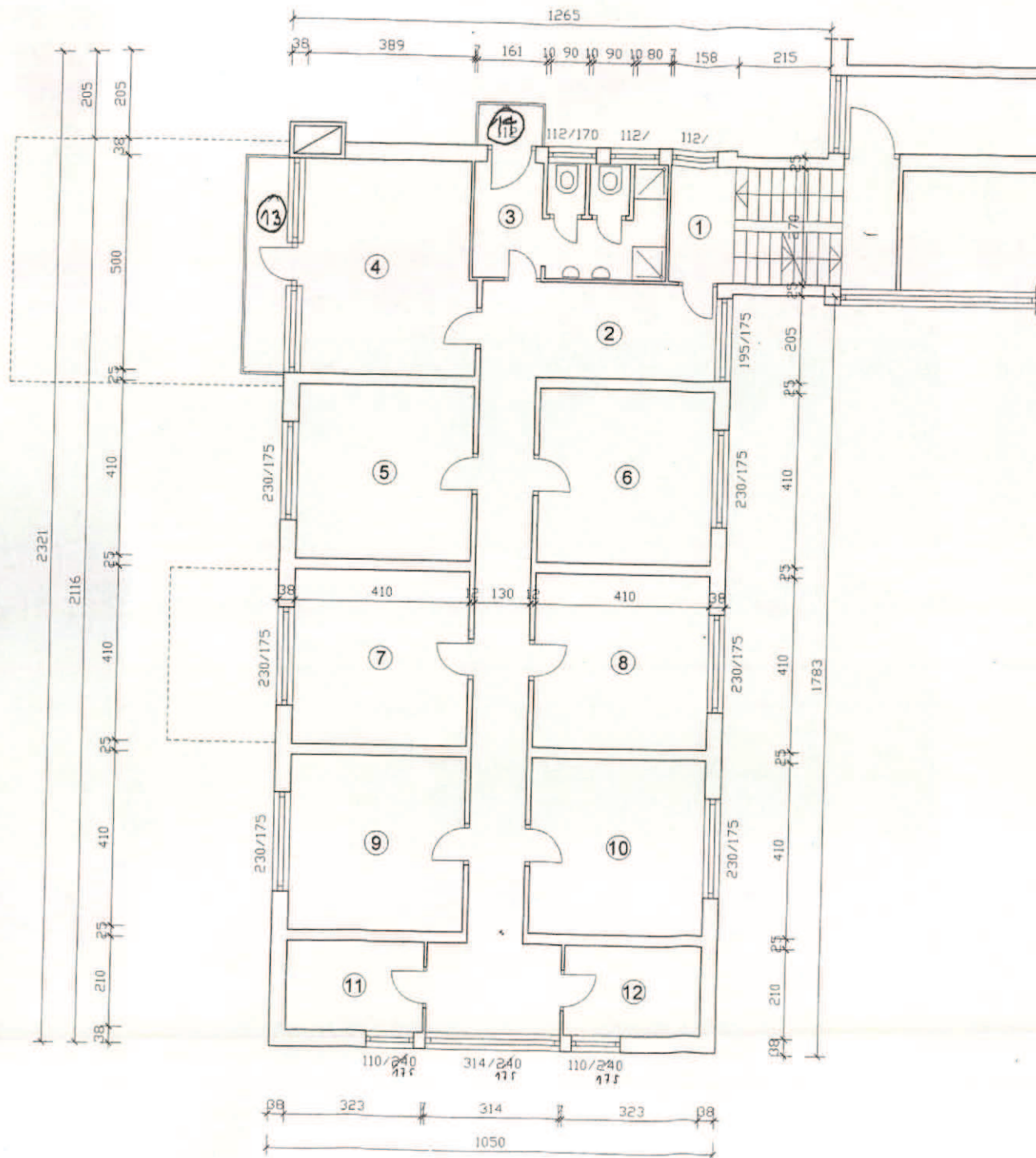
Postojeće stanje Tlocrt 3. kata M1:100
