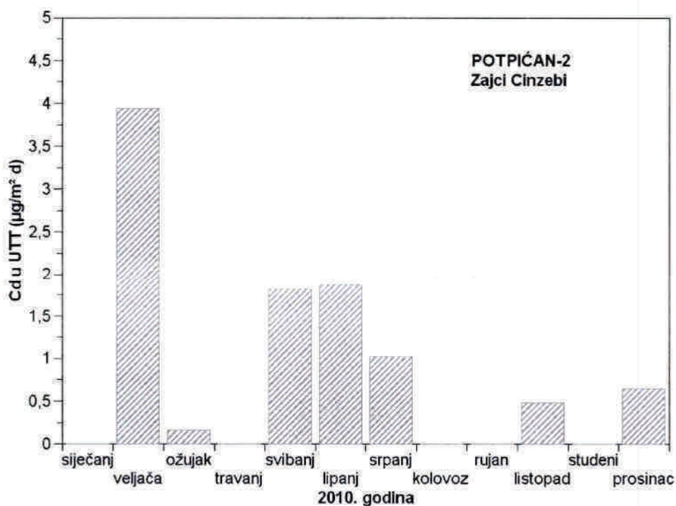
Slika 13 - Srednje mjesečne količine kadmija u ukupnoj taložnoj tvari na mjernoj postaji Potpićan-2 tijekom 2010. godine
