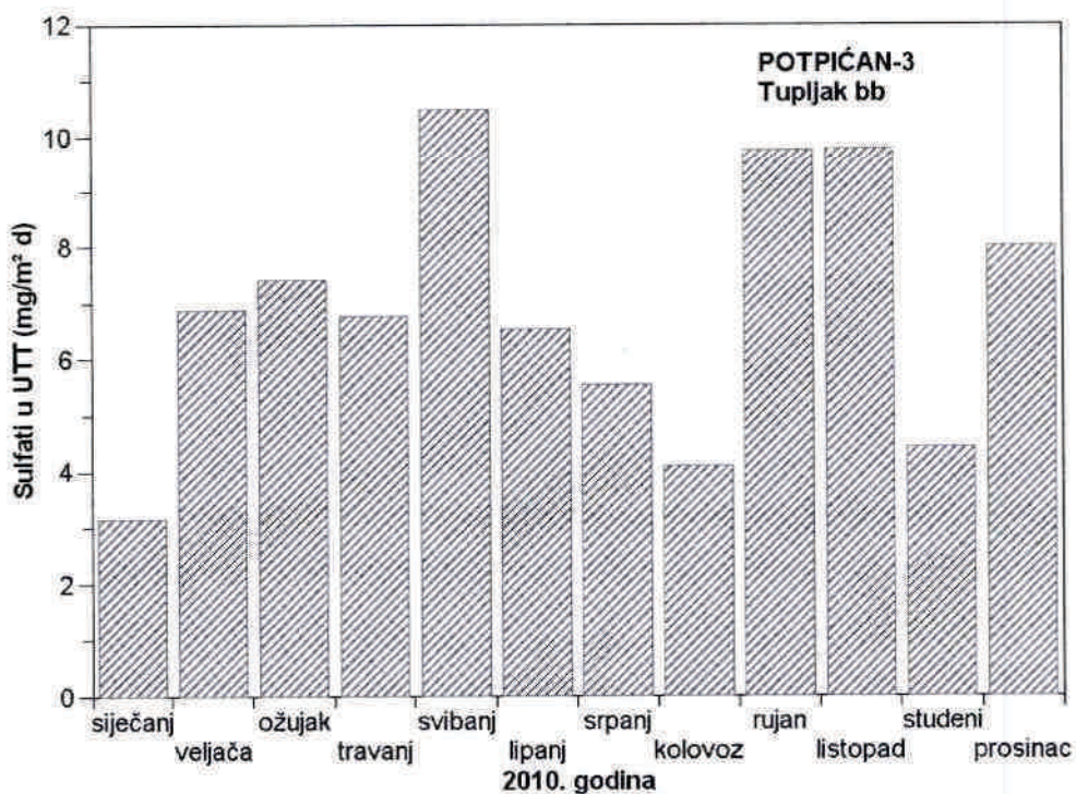
Slika 30 - Srednje mjesečne količine sulfata u ukupnoj taložnoj tvari na mjernoj postaji Potpićan-3 tijekom 2010. godine
