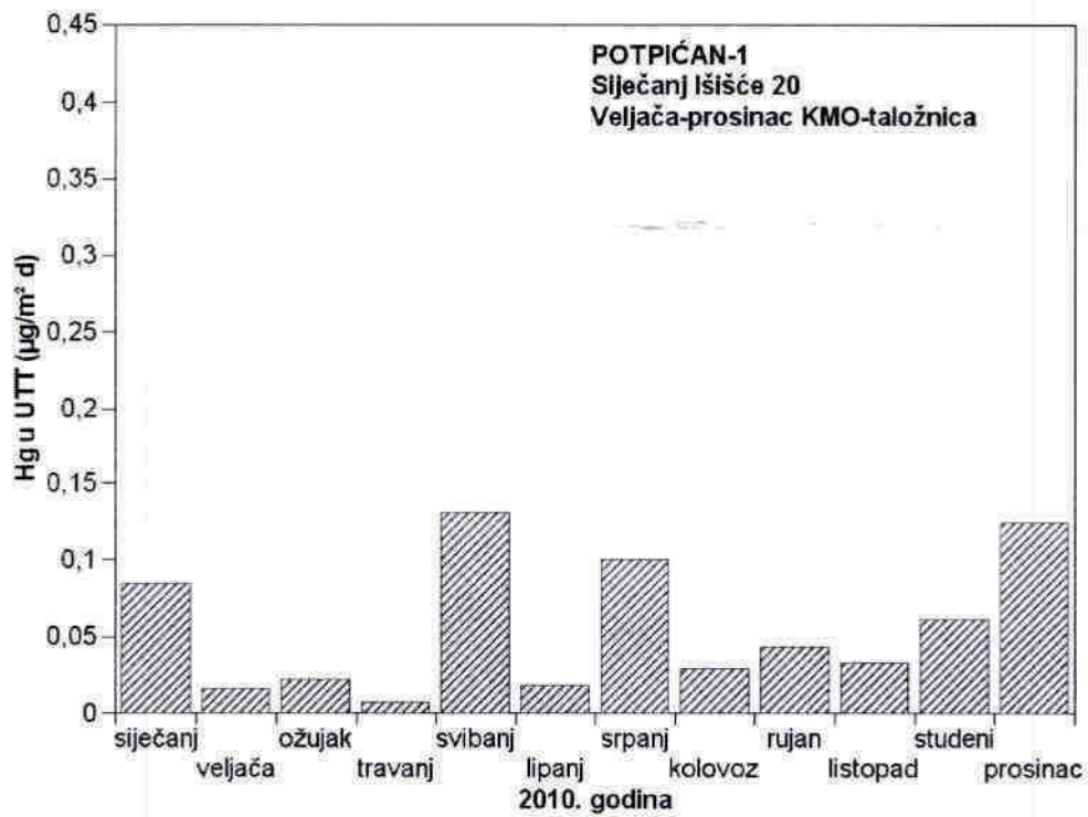
Slika 7 - Srednje mjesečne količine žive u ukupnoj taložnoj tvari na mjernoj postaji Potpićan-1 tijekom 2010. godine
