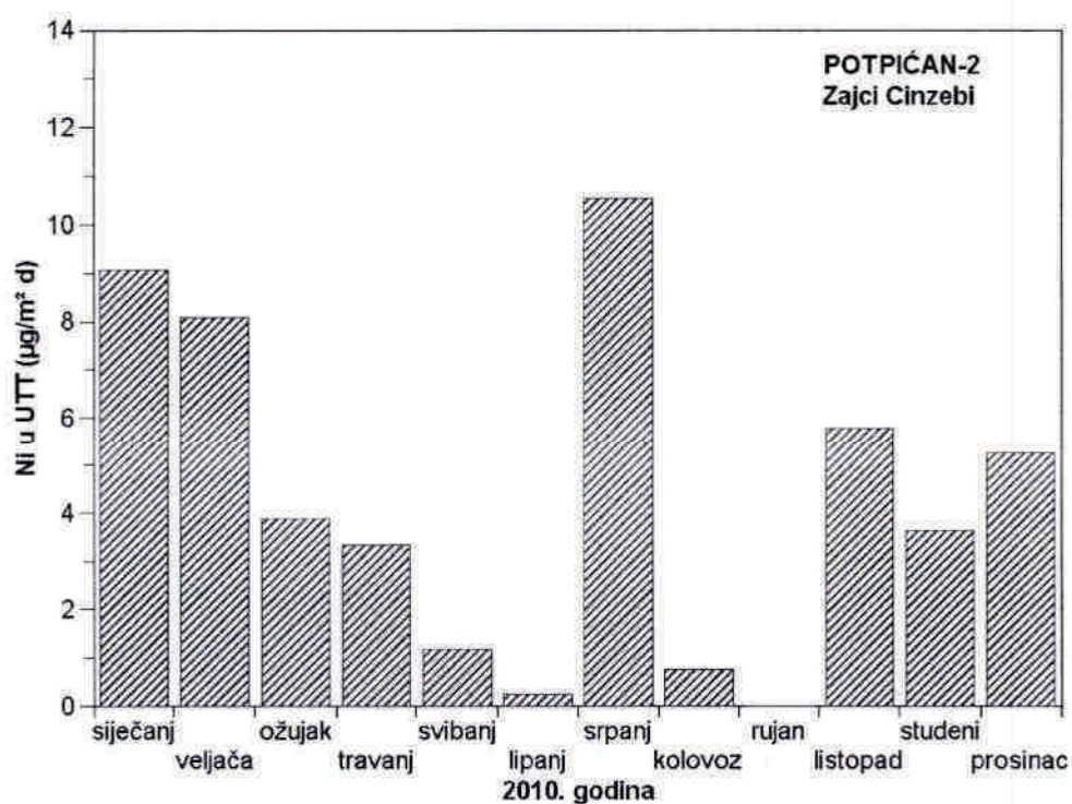
Slika 15 - Srednje mjesečne količine nikla u ukupnoj taložnoj tvari na mjernoj postaji Potpićan-2 tijekom 2010. godine
