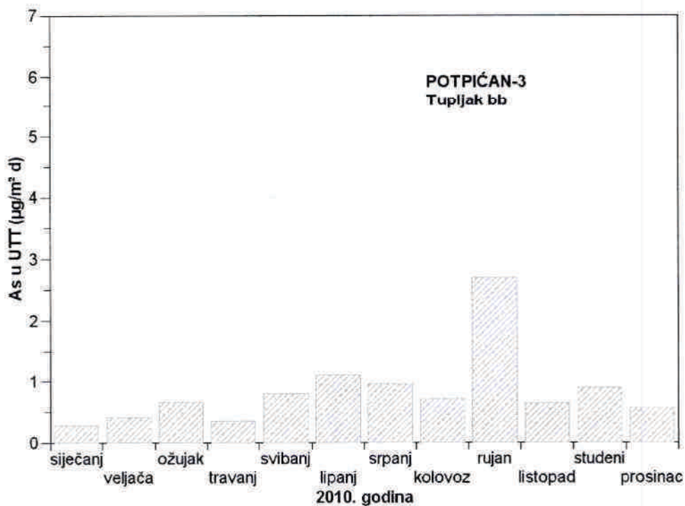
Slika 26 - Srednje mjesečne količine arsena u ukupnoj taložnoj tvari na mjernoj postaji Potpićan-3 tijekom 2010. godine
