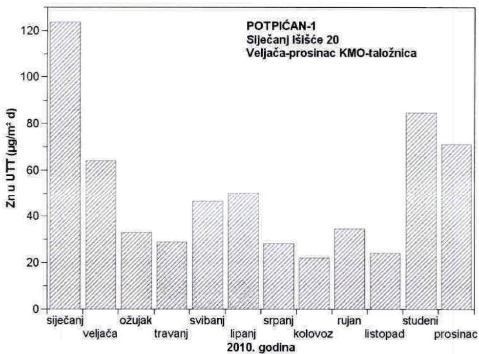
Slika 9 - Srednje mjesečne količine cinka u ukupnoj taložnoj tvari na mjernoj postaji Potpićan-1 tijekom 2010. godine
