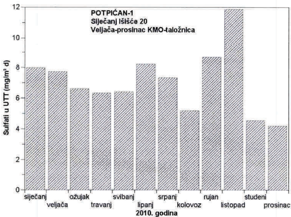
Slika 10 - Srednje mjesečne količine sulfata u ukupnoj taložnoj tvari na mjernoj postaji Potpićan-1 tijekom 2010. godine
