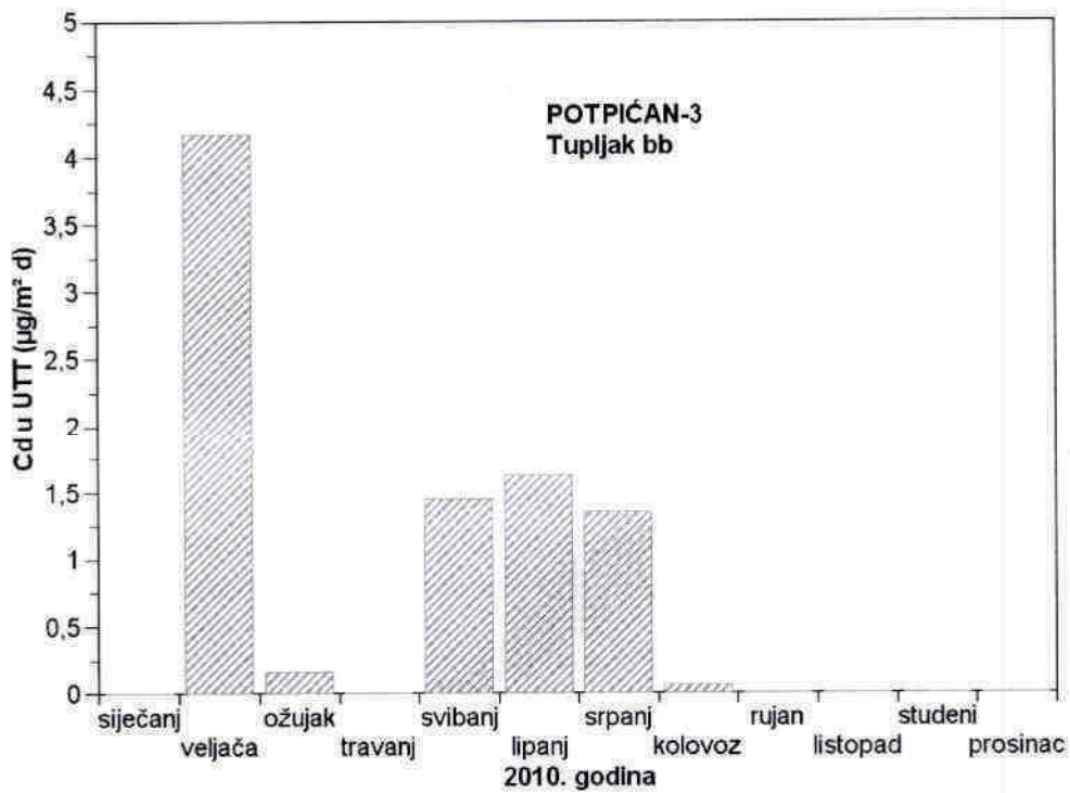
Slika 23 - Srednje mjesečne količine kadmija u ukupnoj taložnoj tvari na mjernoj postaji Potpićan-3 tijekom 2010. godine
