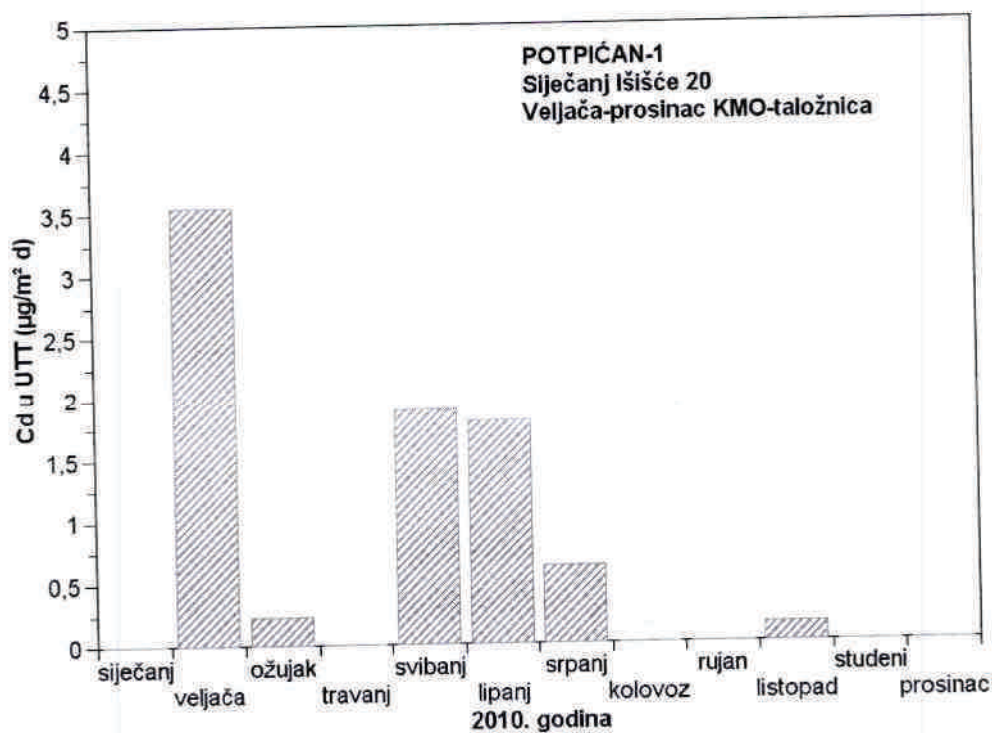
Slika 3 - Srednje mjesečne količine kadmija u ukupnoj taložnoj tvari na mjernoj postaji Potpićan-1 tijekom 2010. godine
