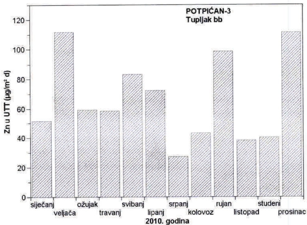
Slika 29 - Srednje mjesečne količine cinka u ukupnoj taložnoj tvari na mjernoj postaji Potpićan-3 tijekom 2010. godine
