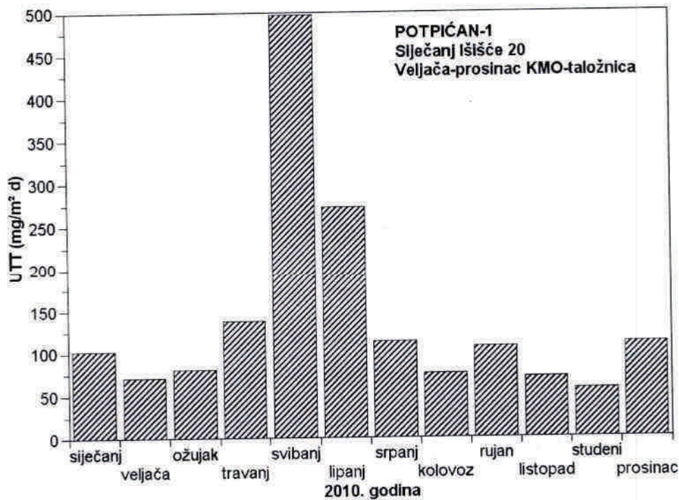
Slika 1 - Srednje mjesečne količine ukupne taložne tvari na mjernoj postaji Potpićan-1 tijekom 2010. godine
