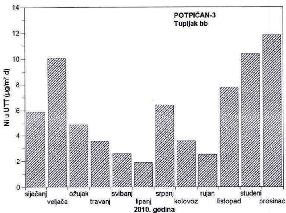
Slika 25 - Srednje mjesečne količine nikla u ukupnoj taložnoj tvari na mjernoj postaji Potpićan-3 tijekom 2010. godine
