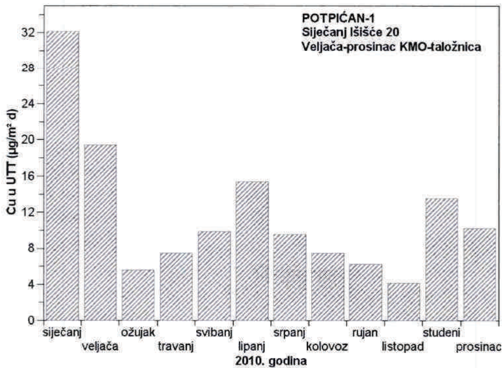
Slika 8 - Srednje mjesečne količine bakra u ukupnoj taložnoj tvari na mjernoj postaji Potpićan-1 tijekom 2010. godine
