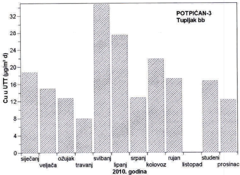
Slika 28 - Srednje mjesečne količine bakra u ukupnoj taložnoj tvari na mjernoj postaji Potpićan-3 tijekom 2010. godine
