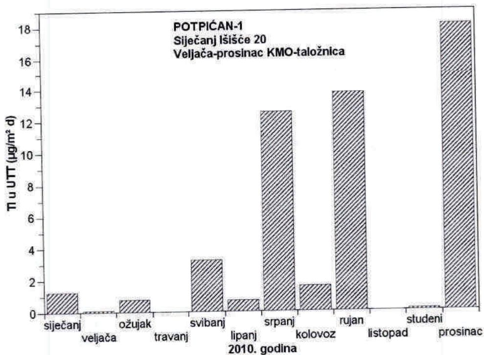
Slika 4 - Srednje mjesečne količine talija u ukupnoj taložnoj tvari na mjernoj postaji Potpićan-1 tijekom 2010. godine
