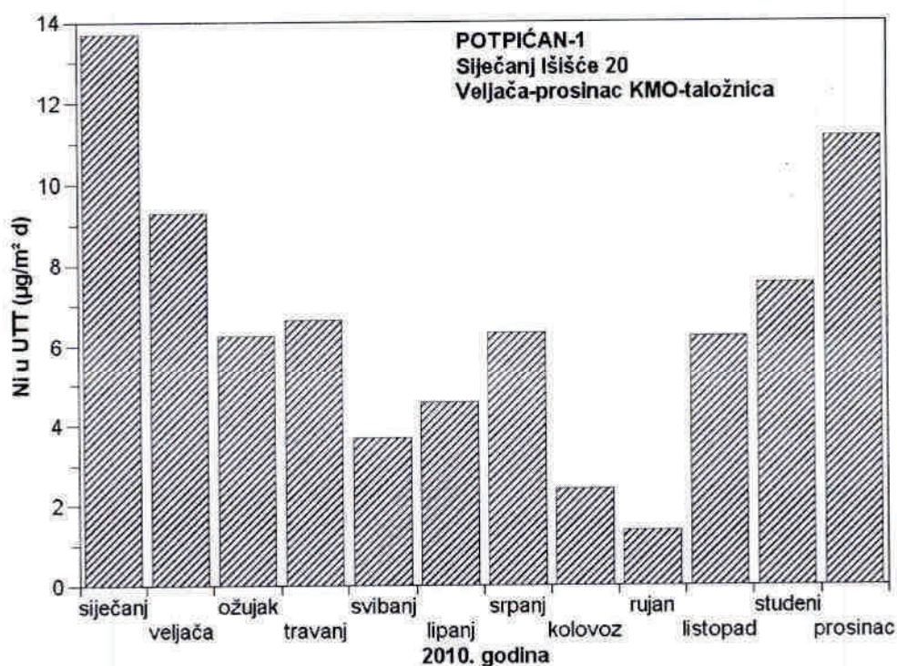
Slika 5 - Srednje mjesečne količine nikla u ukupnoj taložnoj tvari na mjernoj postaji Potpićan-1 tijekom 2010. godine
