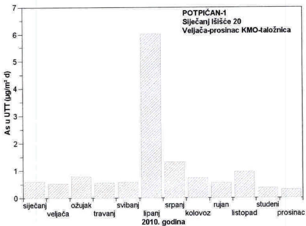
Slika 6 - Srednje mjesečne količine arsena u ukupnoj taložnoj tvari na mjernoj postaji Potpićan-1 tijekom 2010. godine
