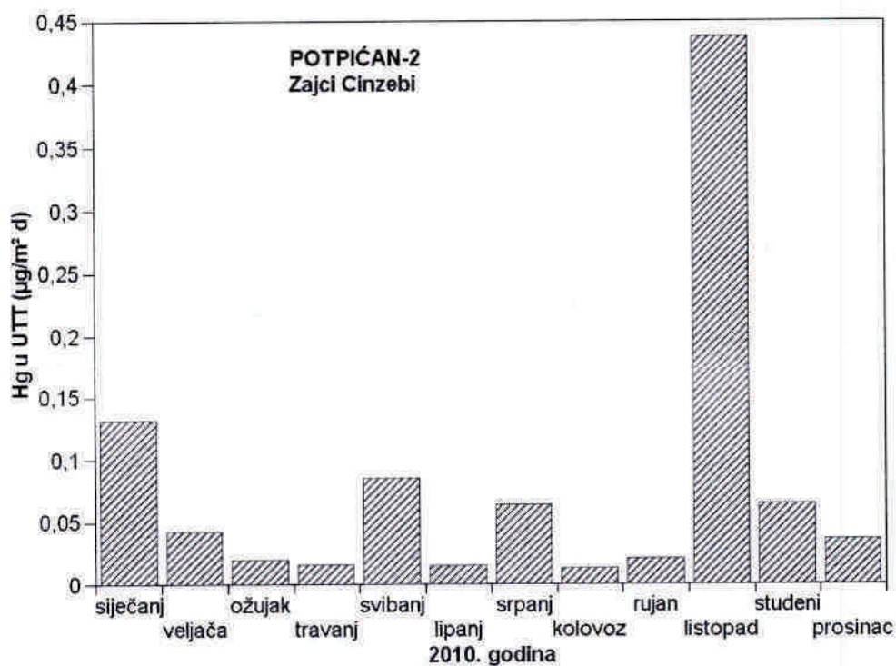
Slika 17 - Srednje mjesečne količine žive u ukupnoj taložnoj tvari na mjernoj postaji Potpićan-2 tijekom 2010. godine
