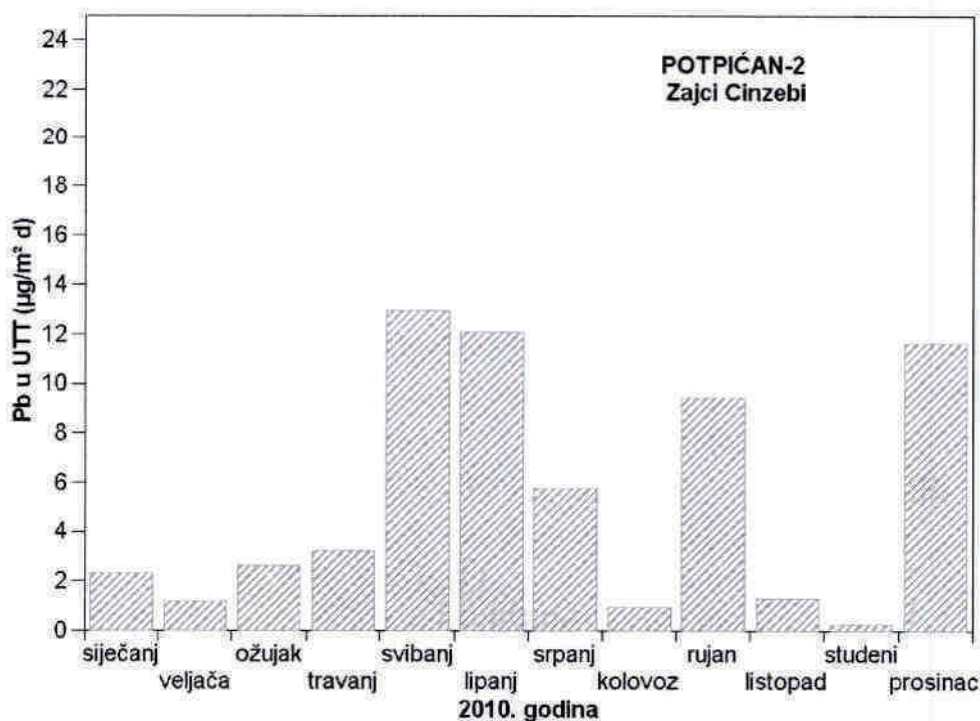
Slika 12 - Srednje mjesečne količine olova u ukupnoj taložnoj tvari na mjernoj postaji Potpićan-2 tijekom 2010. godine
