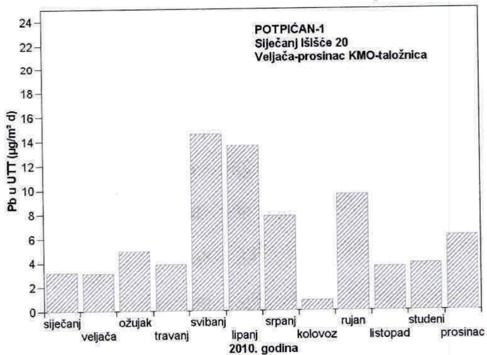
Slika 2 - Srednje mjesečne količine olova u ukupnoj taložnoj tvari na mjernoj postaji Potpićan-1 tijekom 2010. godine
