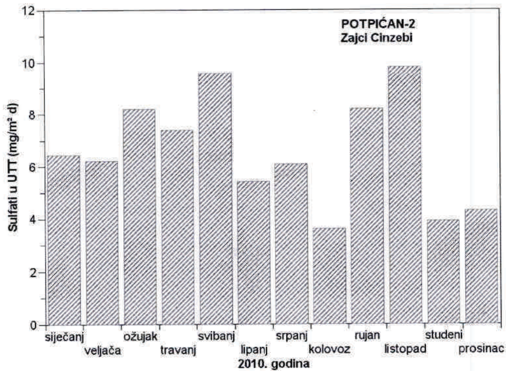
Slika 20 - Srednje mjesečne količine sulfata u ukupnoj taložnoj tvari na mjernoj postaji Potpićan-2 tijekom 2010. godine
