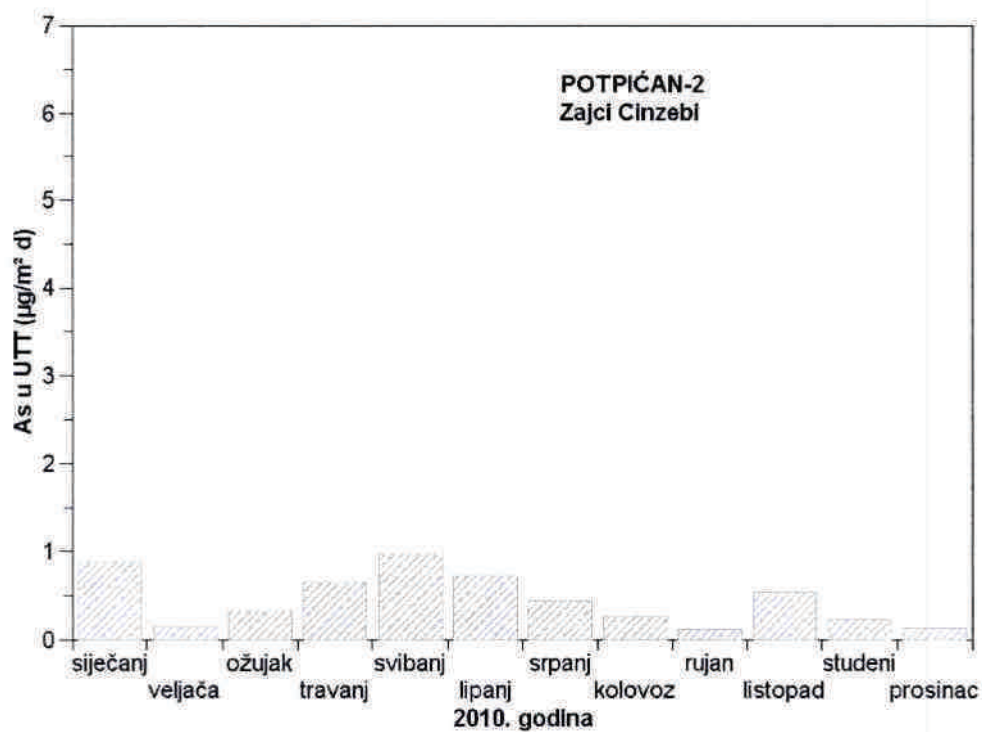
Slika 16 - Srednje mjesečne količine arsena u ukupnoj taložnoj tvari na mjernoj postaji Potpićan-2 tijekom 2010. godine
