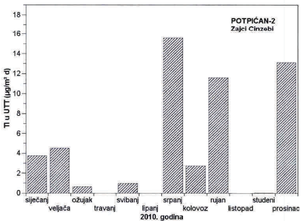
Slika 14 - Srednje mjesečne količine talija u ukupnoj taložnoj tvari na mjernoj postaji Potpićan-2 tijekom 2010. godine
