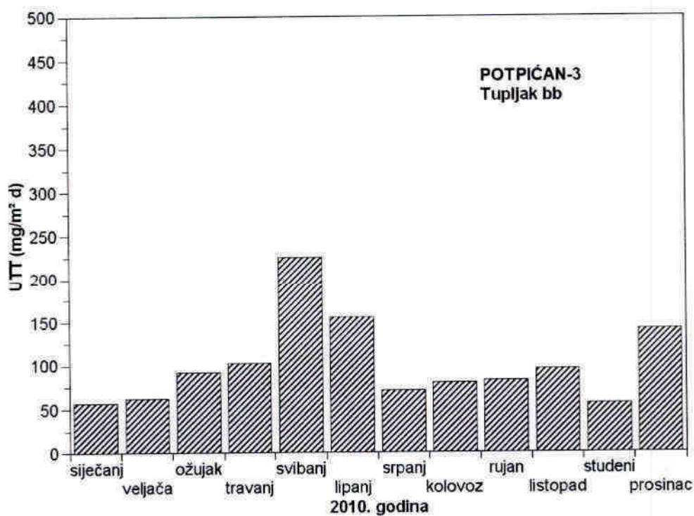
Slika 21 - Srednje mjesečne količine ukupne taložne tvari na mjernoj postaji Potpićan-3 tijekom 2010. godine
