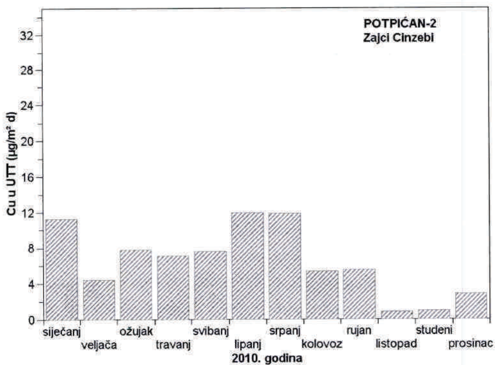
Slika 18 - Srednje mjesečne količine bakra u ukupnoj taložnoj tvari na mjernoj postaji Potpićan-2 tijekom 2010. godine
