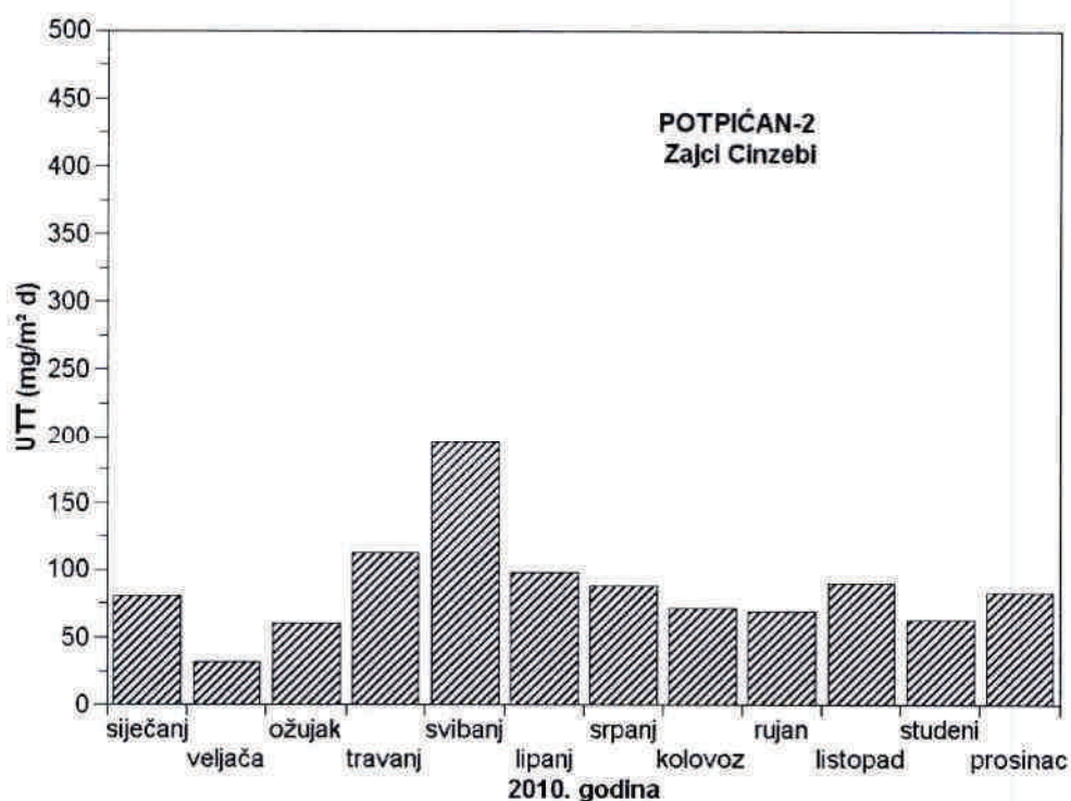
Slika 11 - Srednje mjesečne količine ukupne taložne tvari na mjernoj postaji Potpićan-2 tijekom 2010. godine
