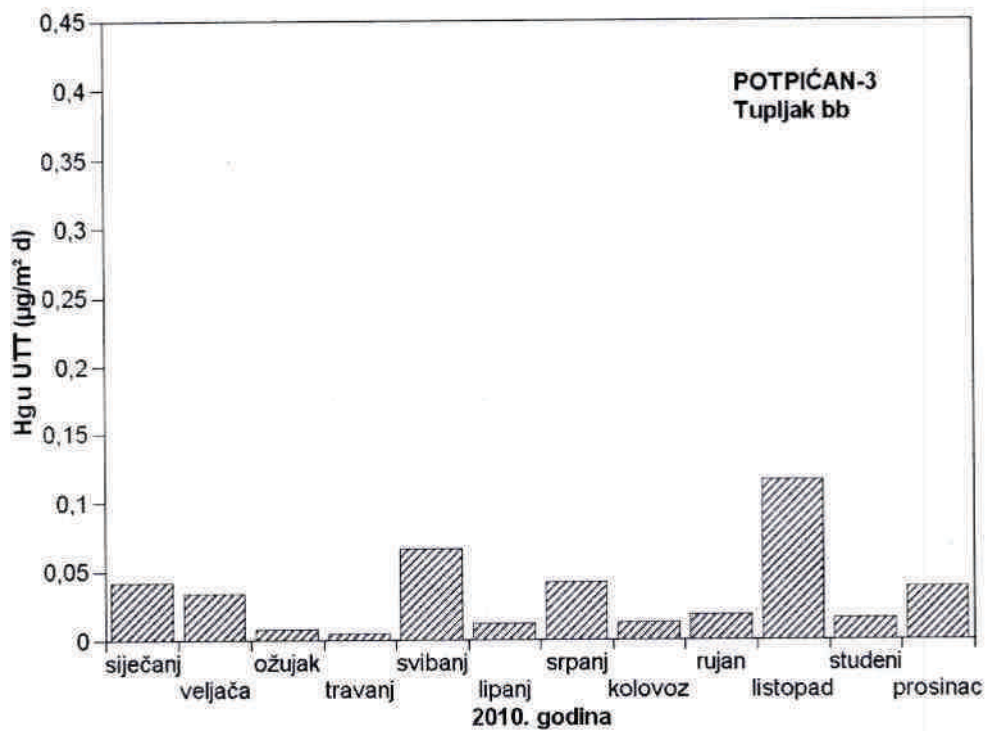
Slika 27 - Srednje mjesečne količine žive u ukupnoj taložnoj tvari na mjernoj postaji Potpićan-3 tijekom 2010. godine
