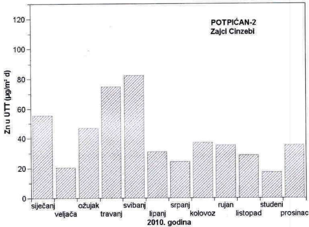
Slika 19 - Srednje mjesečne količine cinka u ukupnoj taložnoj tvari na mjernoj postaji Potpićan-2 tijekom 2010. godine
