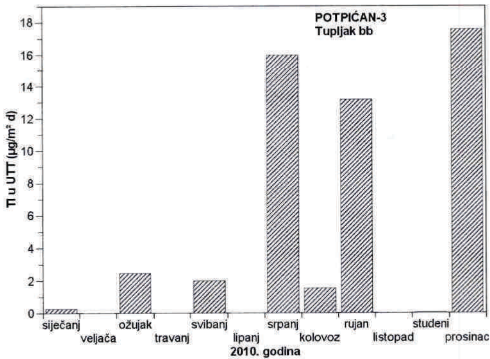
Slika 24 - Srednje mjesečne količine talija u ukupnoj taložnoj tvari na mjernoj postaji Potpićan-3 tijekom 2010. godine
