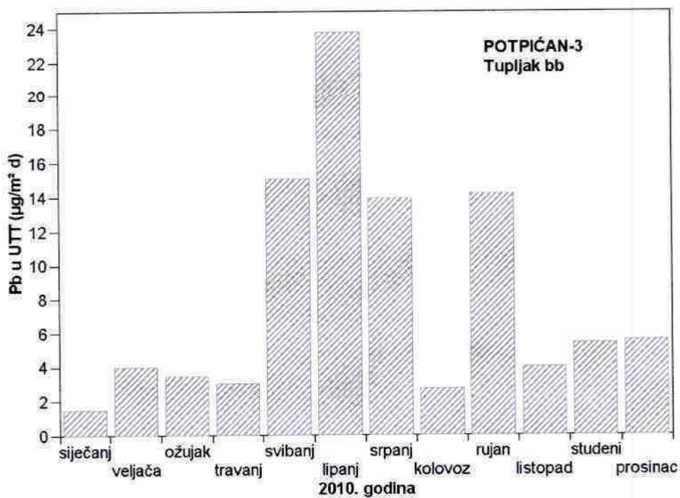
Slika 22 - Srednje mjesečne količine olova u ukupnoj taložnoj tvari na mjernoj postaji Potpićan-3 tijekom 2010. godine
